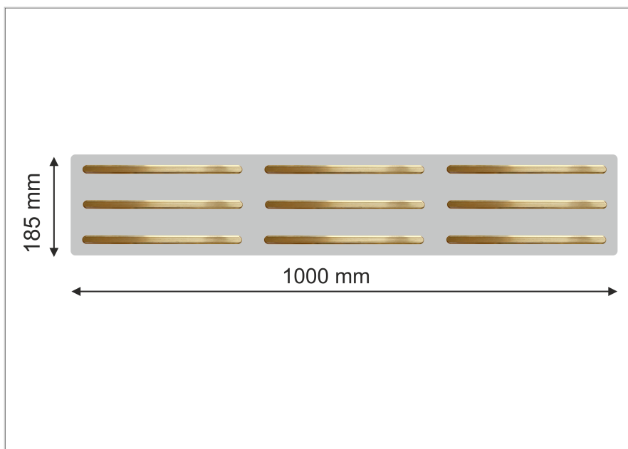
Schematische Darstellung - neun Messingleitlinien auf Trägermaterial (MS 1000)
