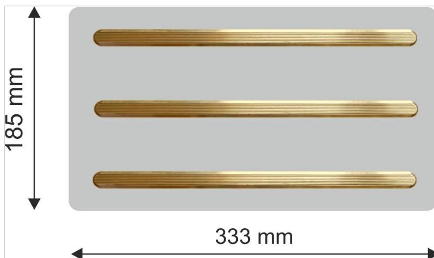
Schematische Darstellung - Messingleitlinien auf Trägermaterial (MS 333)
