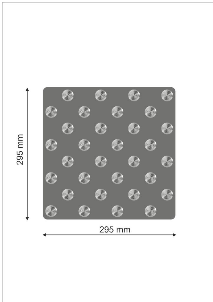
Schematische Darstellung - Edelstahlnoppen auf Trägermaterial (EST 295)
