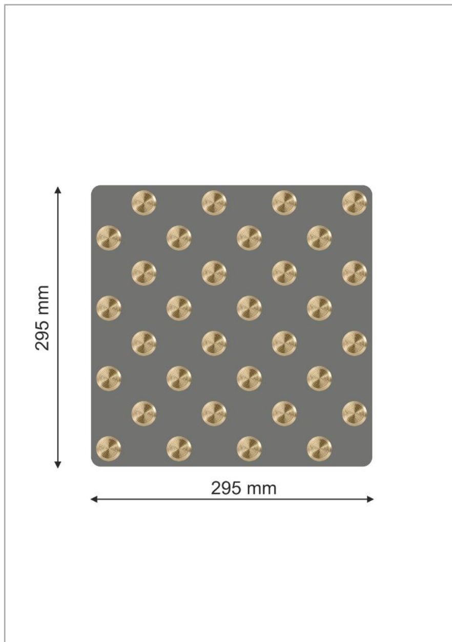
Schematische Darstellung - Messingnoppen auf Trägermaterial (MS 295)
