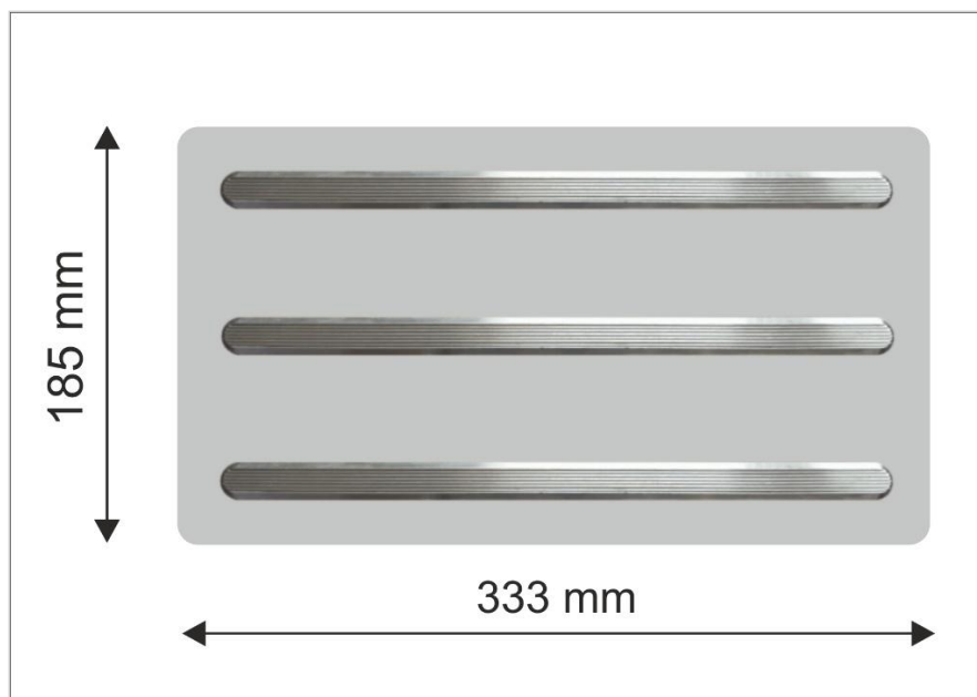
Schematische Darstellung - Edelstahlleitlinien auf Trägermaterial (EST 333)
