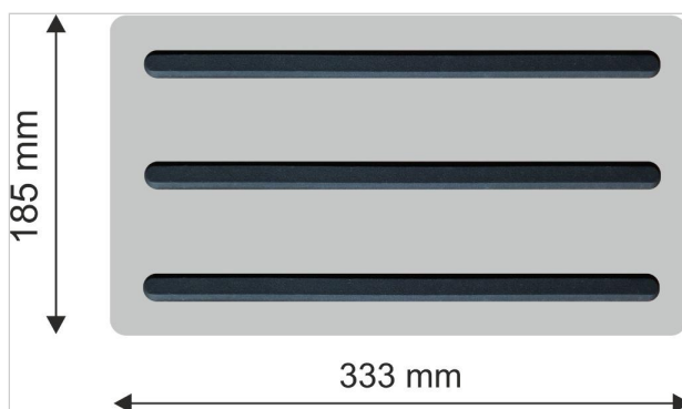
Schematische Darstellung - Taktile Kunststoffleitlinien aus TPU auf Trägermaterial (TPU 333)
